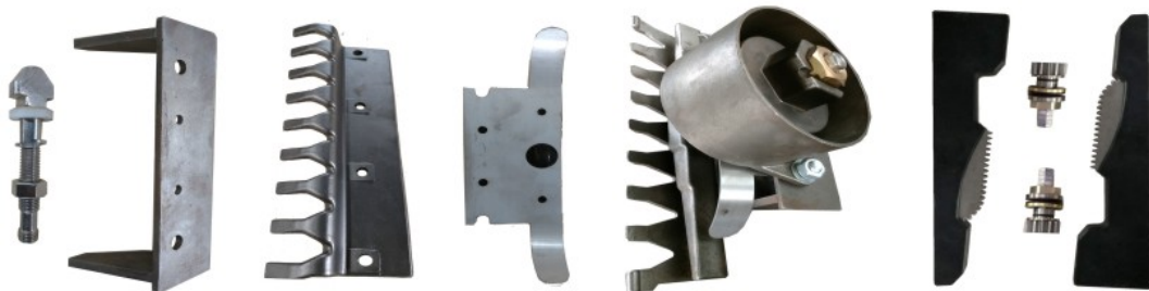
振动筛配件 Shale Shaker Parts
