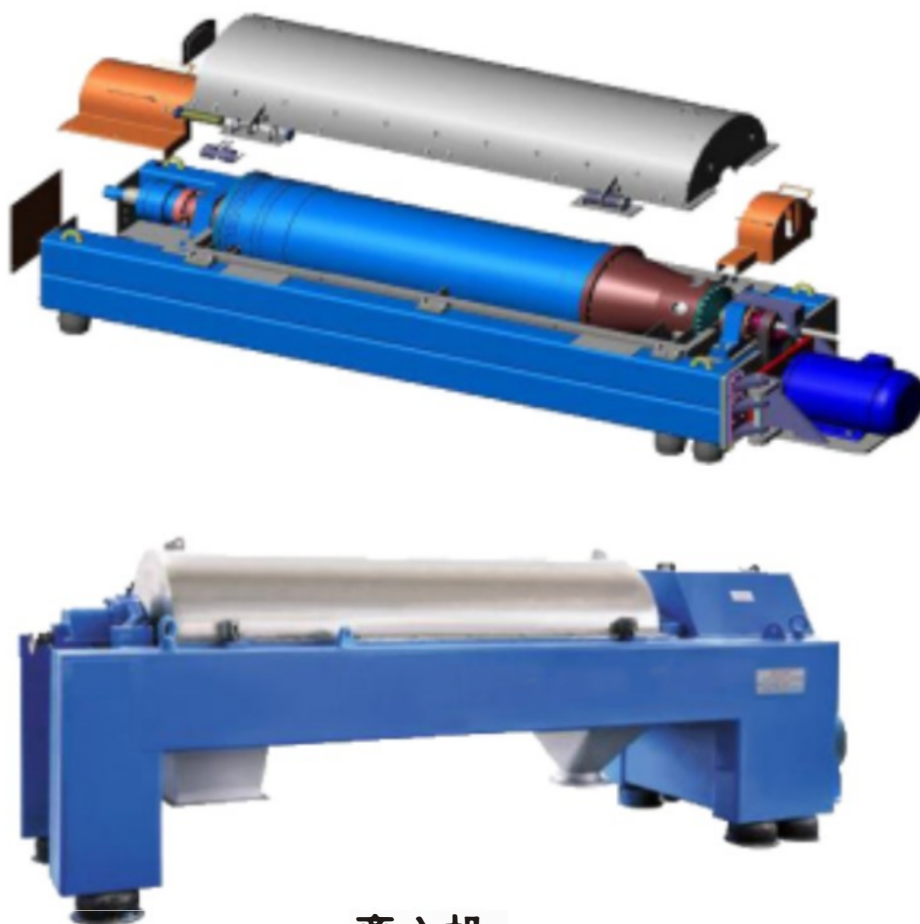
■离心机 Decanter Centrifuge
