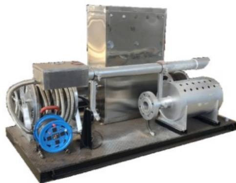
■ 电子点火装置 Flare Ignition Device
