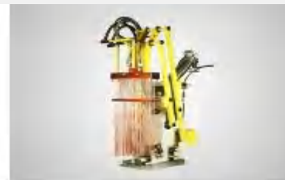
四连杆喷雾机 FOUR-BAR SPRAYER W/S
